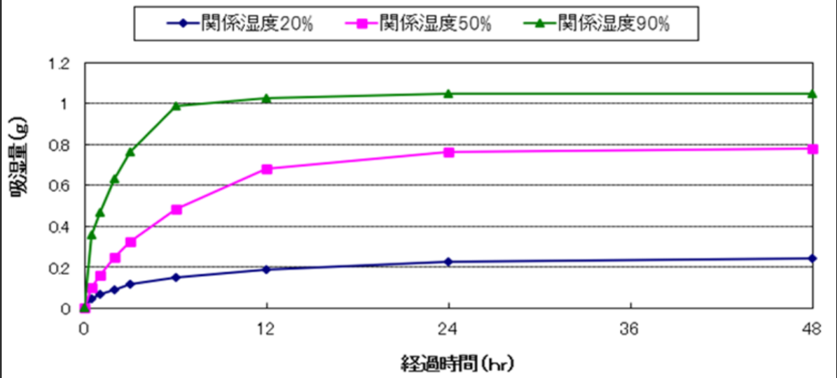
アブリオAW400 吸湿量(g)の時間変化(25℃・10×10cmあたり)
